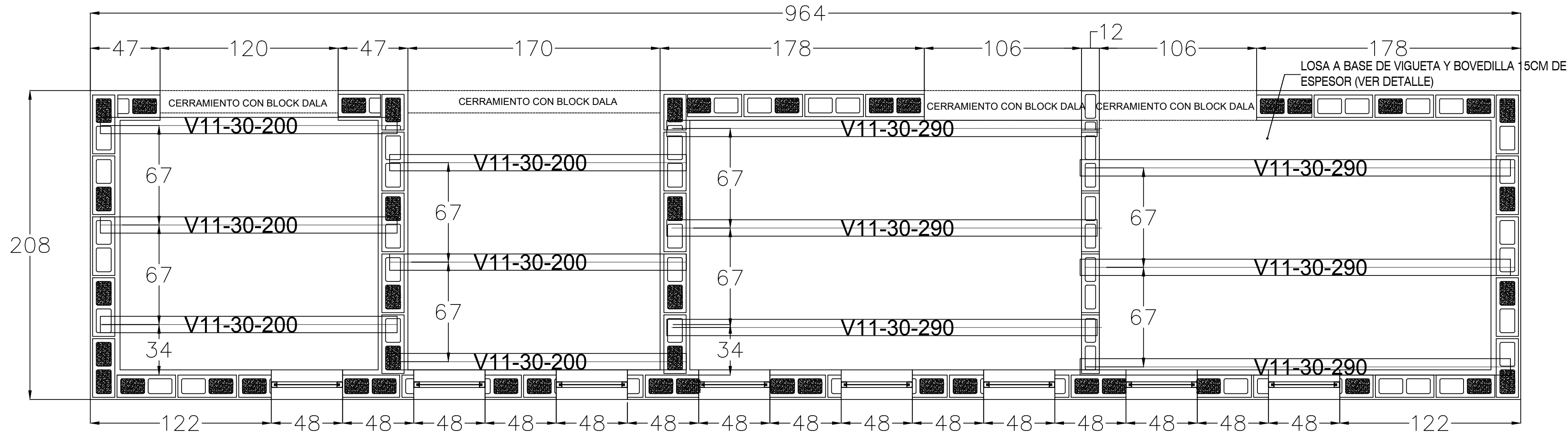
PLANTA ESTRUCTURAL DE AZOTEA MÓDULO DE BAÑOS PLANTA
