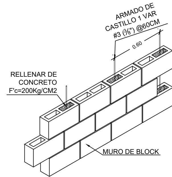
DETALLE TIPO DE REFUERZO PARA MURO DE BLOCK ISOMETRICO ESCALA 1:20
