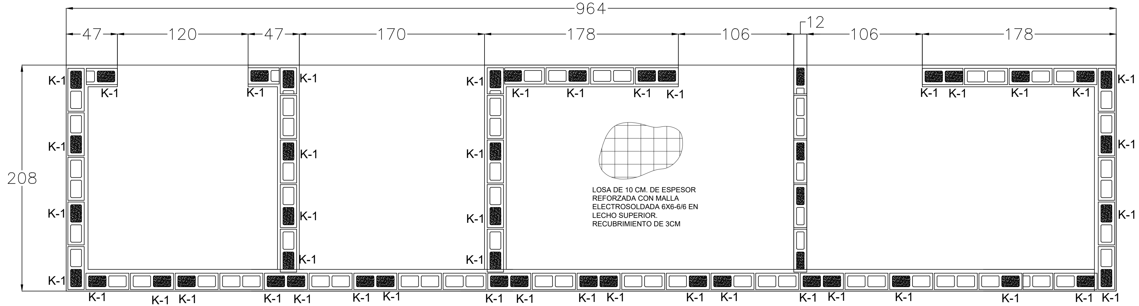
CIMENTACIÓN MÓDULO DE BAÑOS PLANTA
