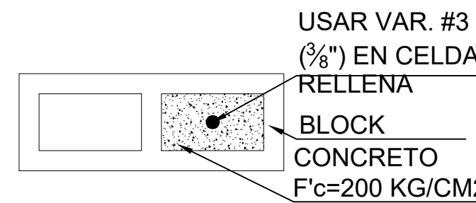
CASTILLO PLANTA K-1 ESC. 1:10
